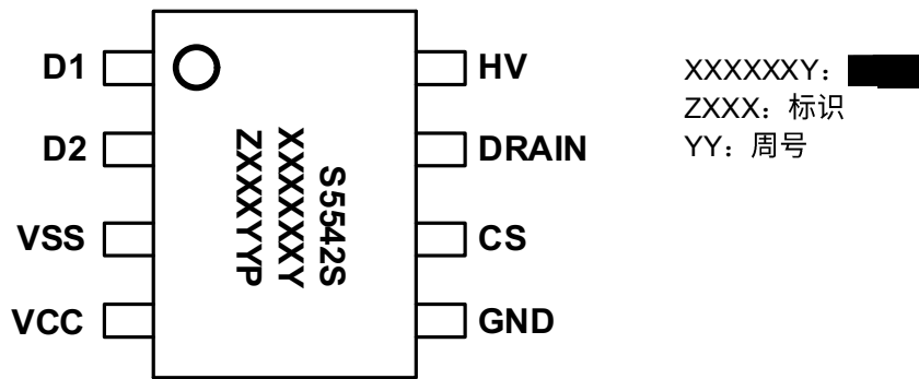
图 7 封装管脚图
