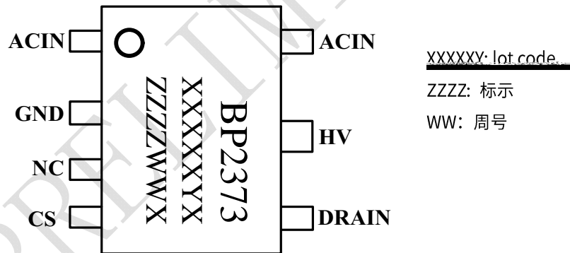
图 2 管脚封装图
